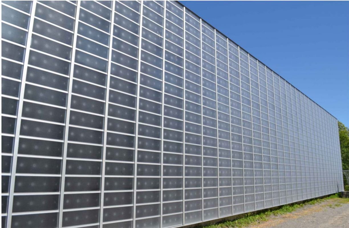
Bild 2: Der Solar-Luftkollektor LUBI TM - preisgekrönter Star der Wärmeeffizienz – wandelt Sonnenenergie über das Medium Luft in Wärme um. Mit einem Wirkungsgrad von über 80 Prozent verfügt LUBI über einen der höchsten Wirkungsgrade, der je für einen Solar-Luftkollektor gemessen wurde. Foto: GoGaS
