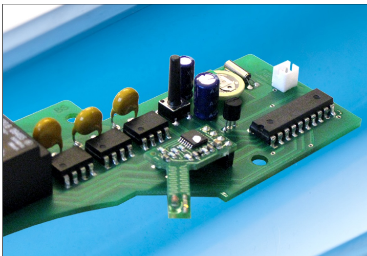
Bild 2: Platine mit Feuchte- und Temperatursensor. Foto: Lunos
