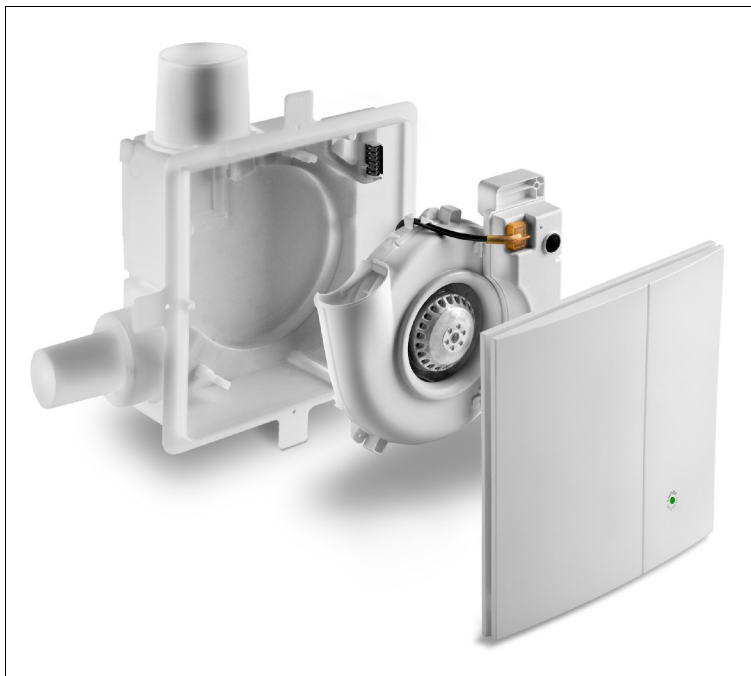
Bild 1: Silvento UP-Gehäuse 3/UP-R mit Zweitraumanschluss 3/S2 und Ventilatoreinsatz V. Foto: Lunos
